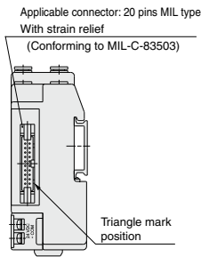
60PG (20 pins)
