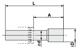
寸法表
