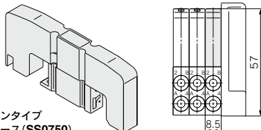
スリムコンパクト 一体形ベース (SS0751)
