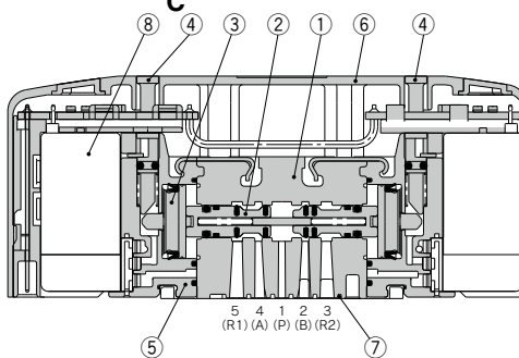
デュアル3ポート弁：S07B0 A C
