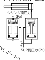
〈チェック弁作動原理図〉
