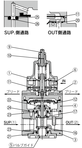
IR3120
