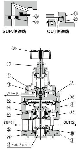
IR3120
