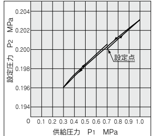
IR3120-03
